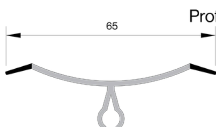
Profilé femelle
